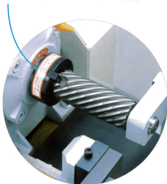
回り止めリング(カッターNo.39以上に使用)
